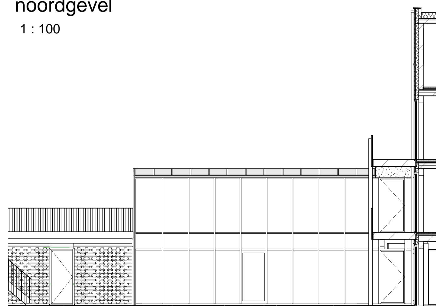
zijgevel kas 1 : 100
