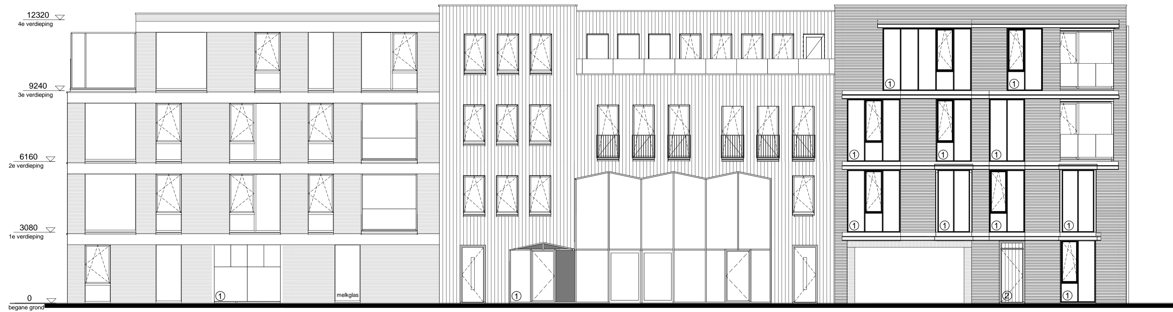
zuidgevel 1 : 100
