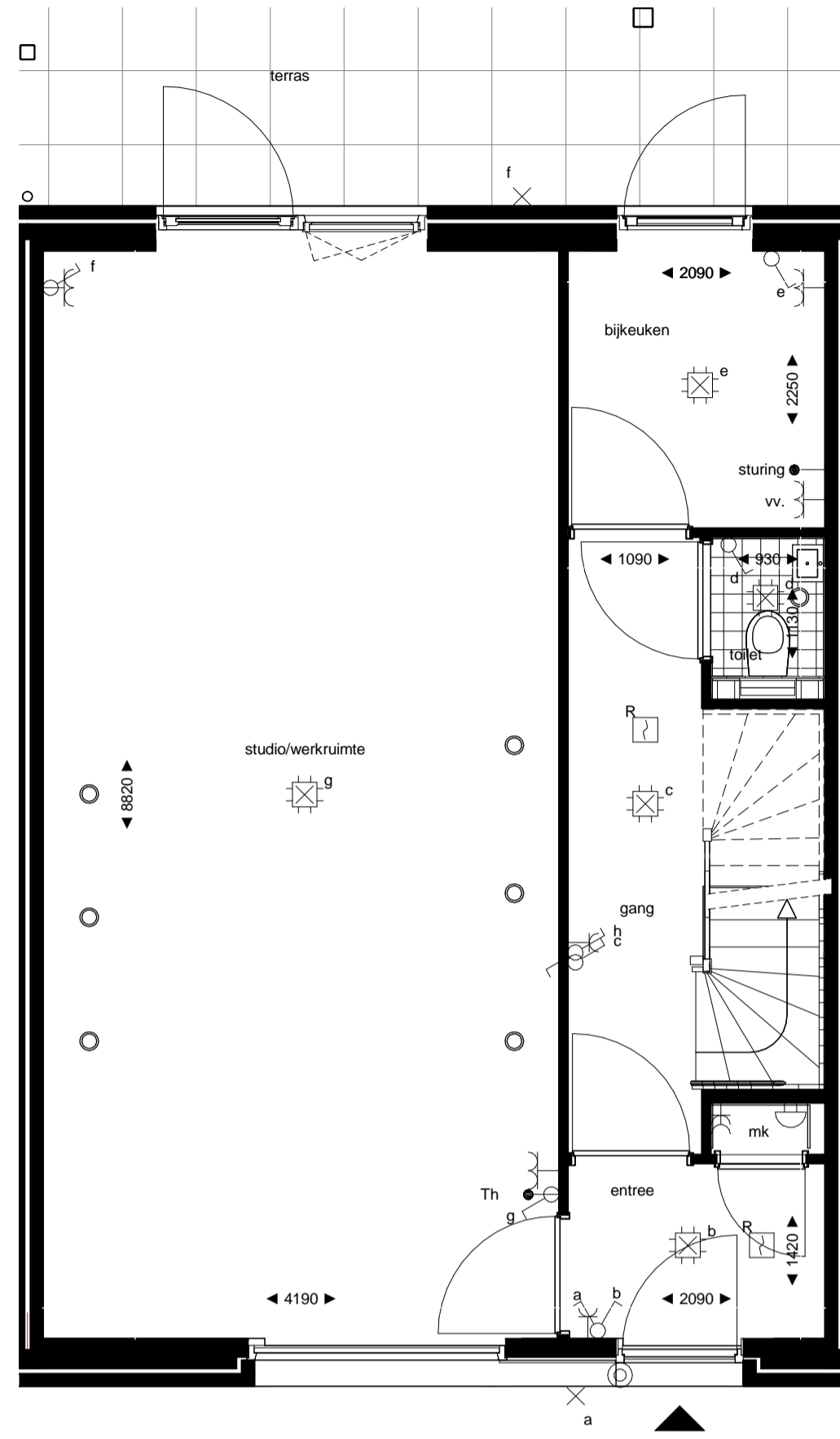
begane grond 1 : 50
