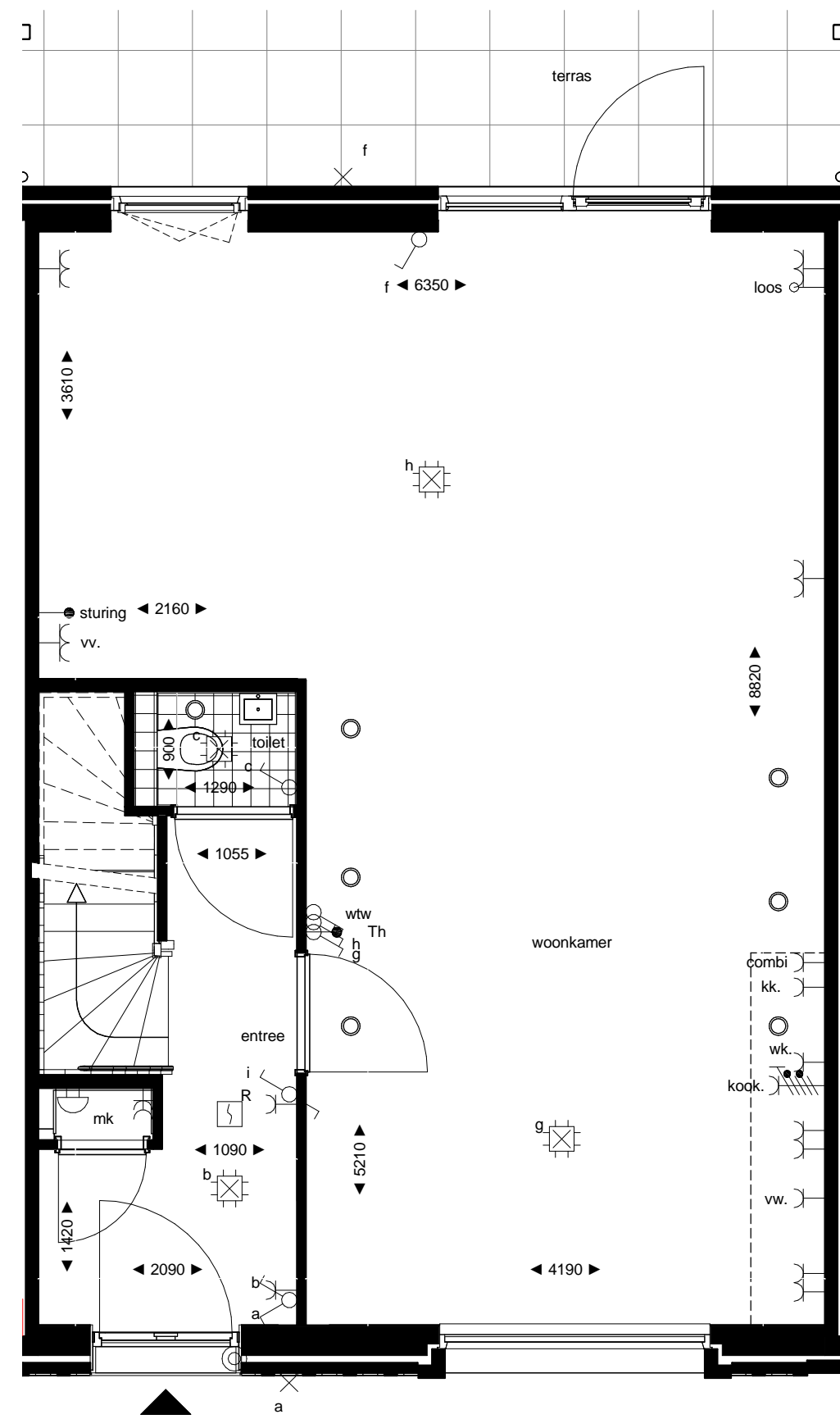
begane grond 1 : 50
