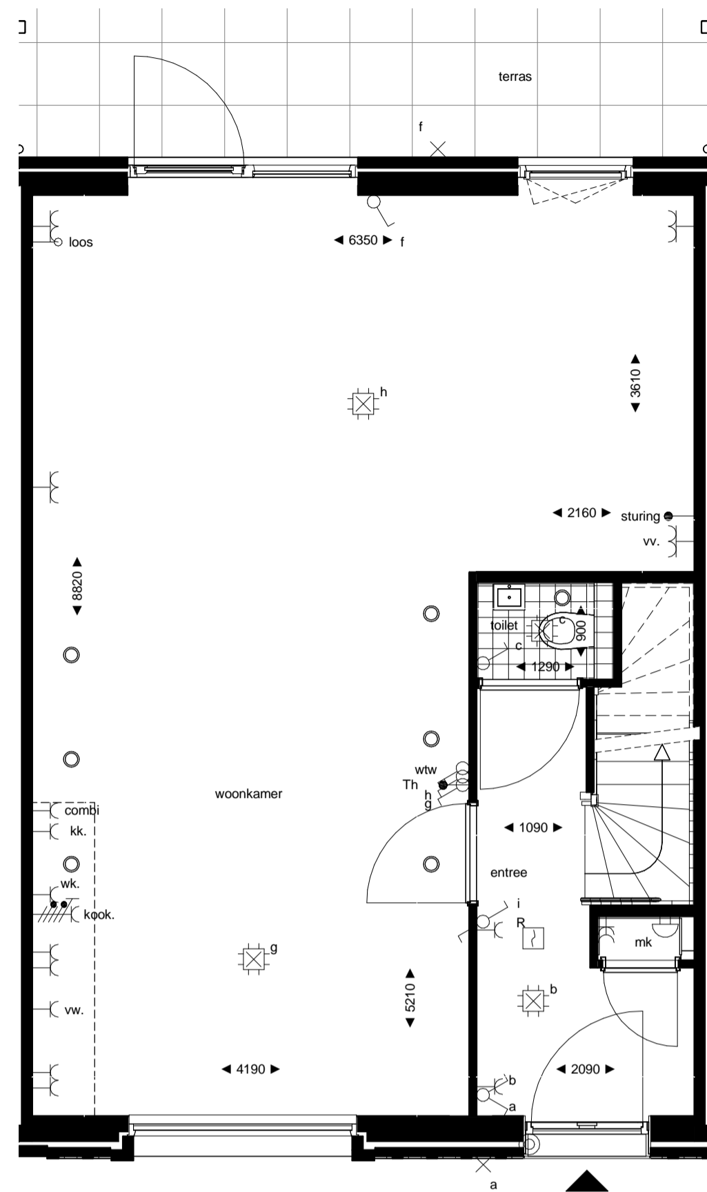
begane grond 1 : 50
