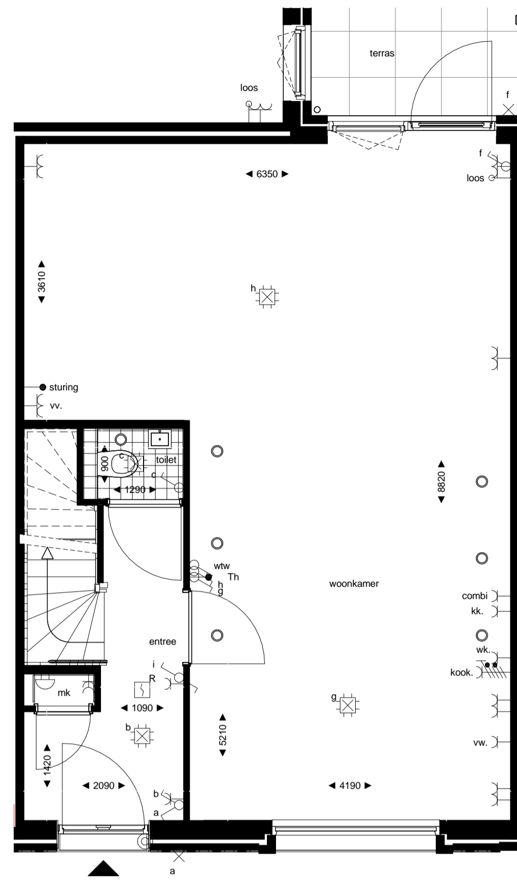
begane grond 1 : 50
