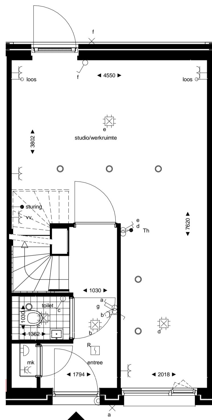
begane grond 1 : 50
