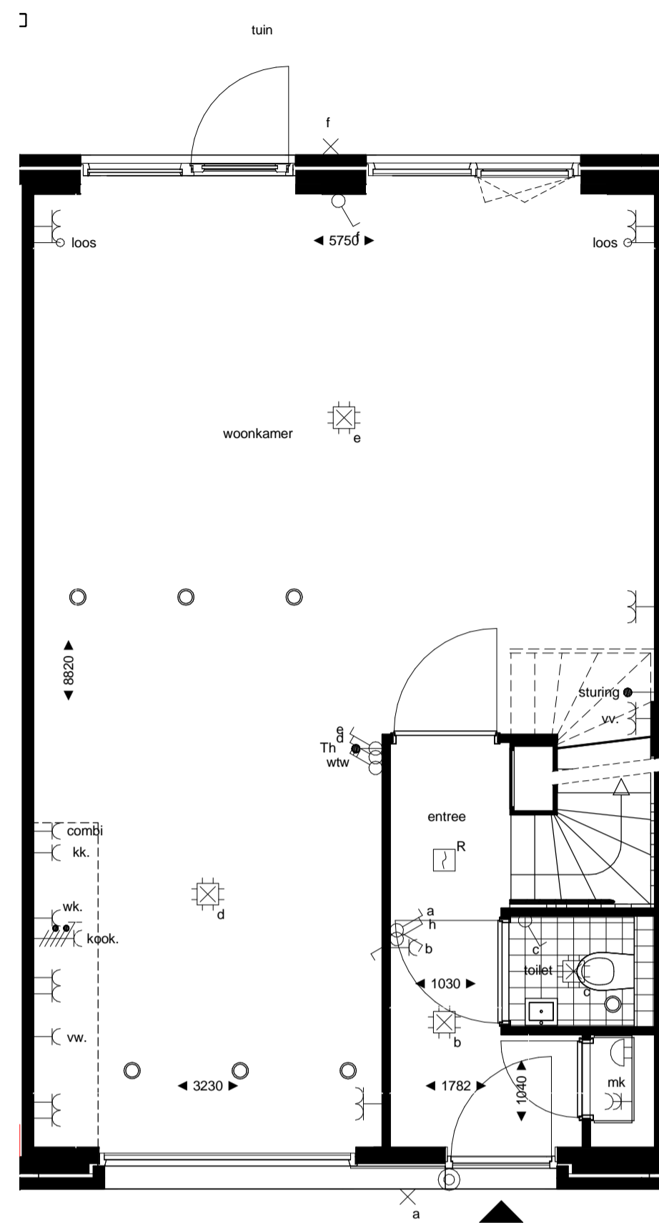
begane grond 1 : 50
