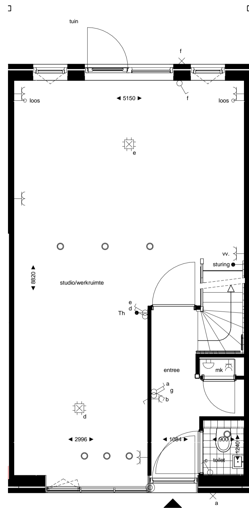
begane grond 1 : 50
