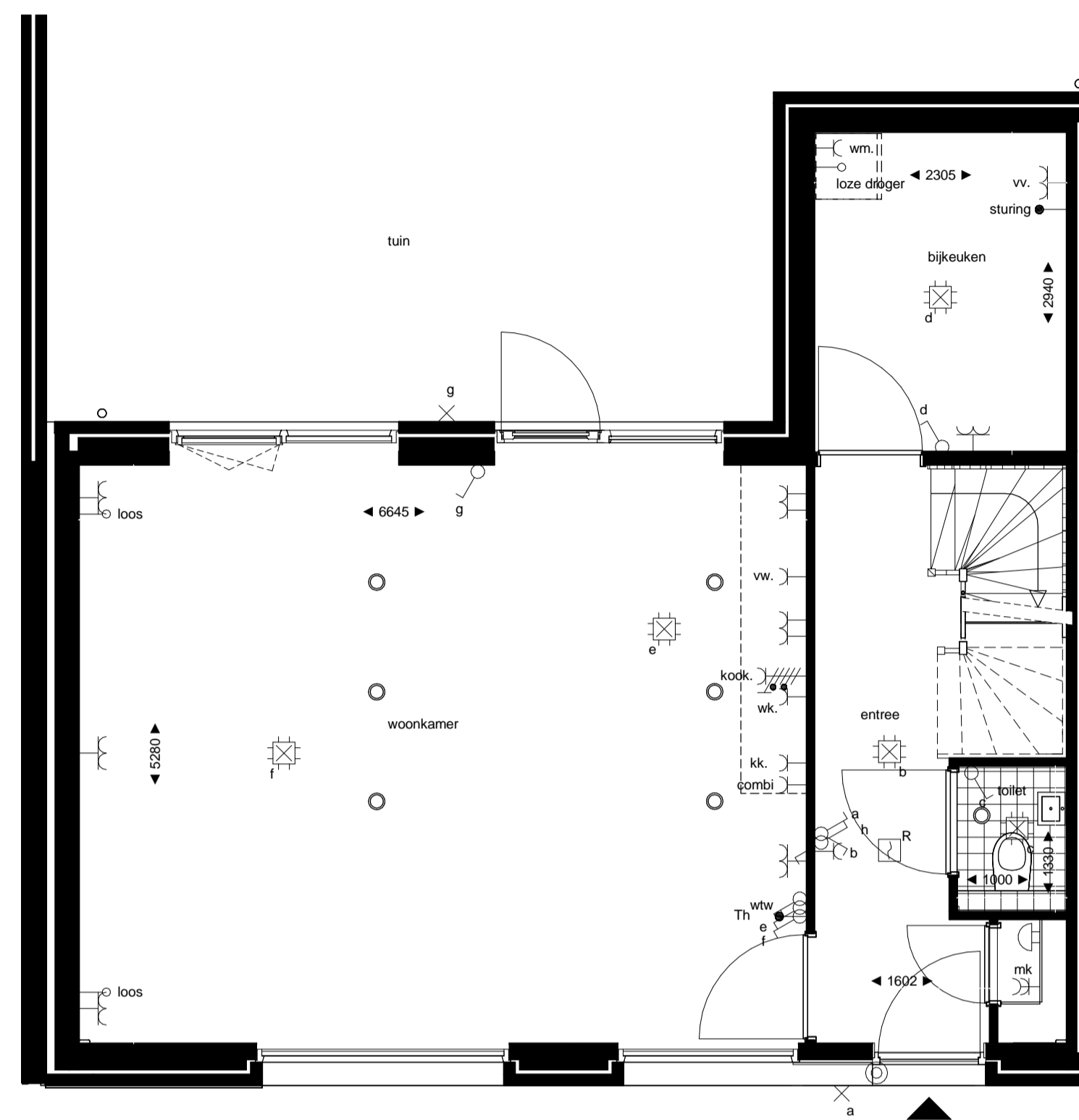
begane grond 1 : 50
