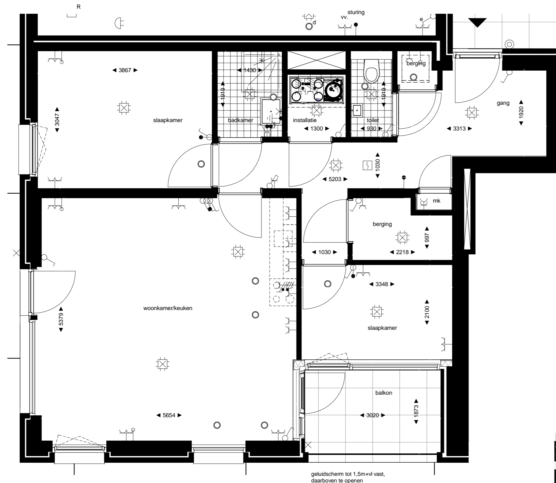
begane grond 1 : 50
