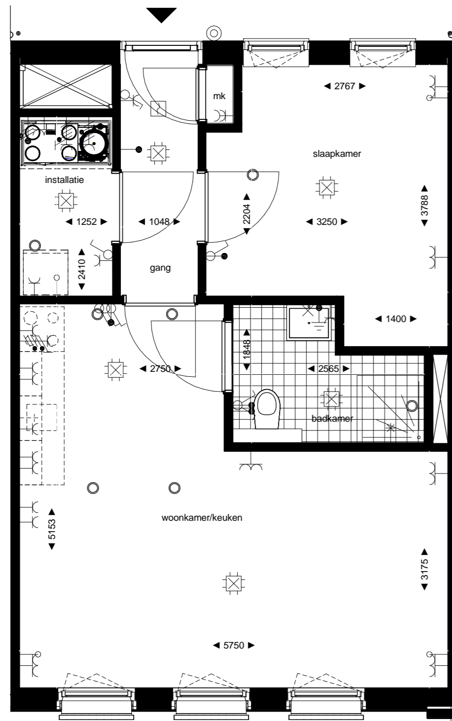
2e verdieping 1 : 50
